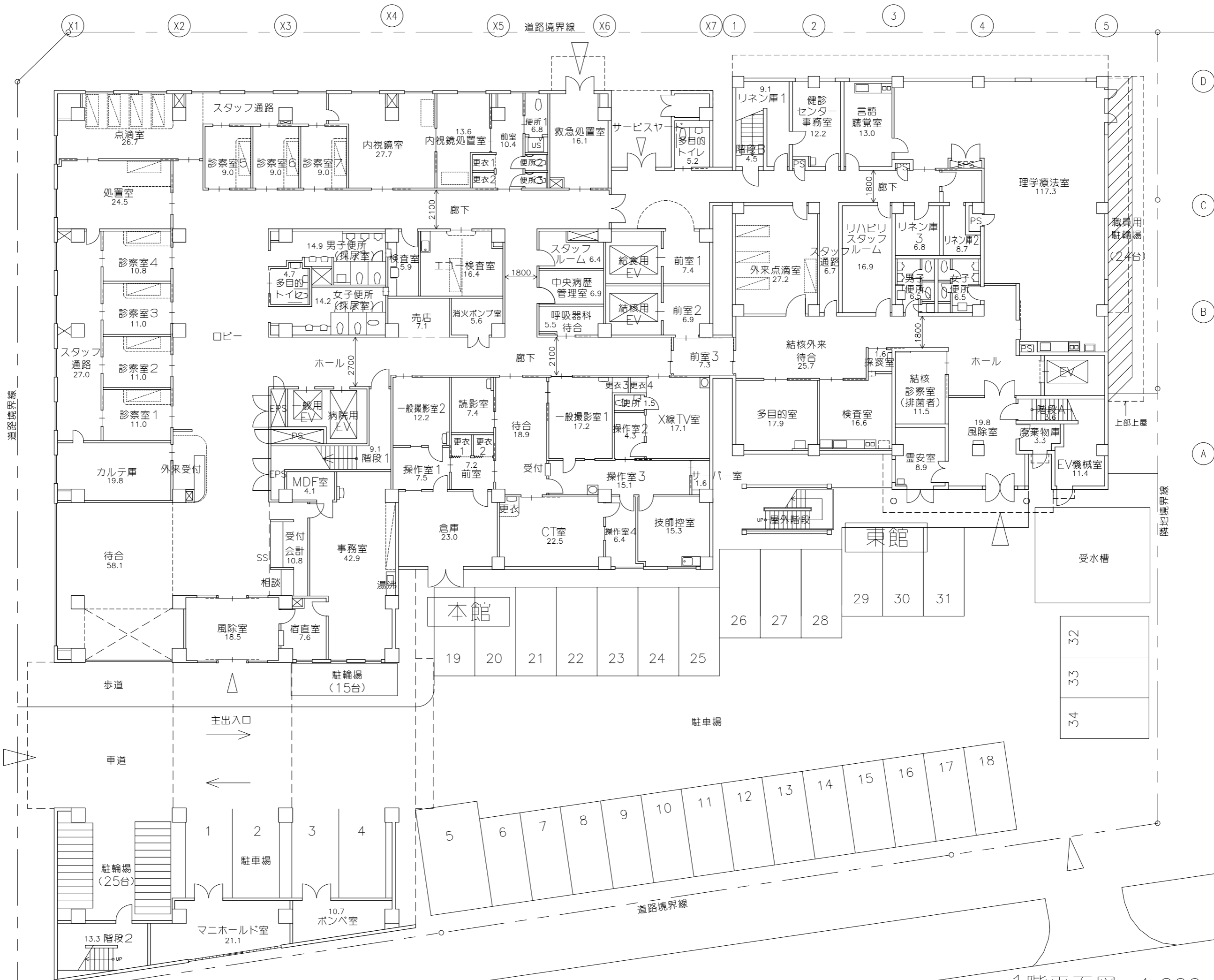
1階平面図 1:200 (A3) 191211
